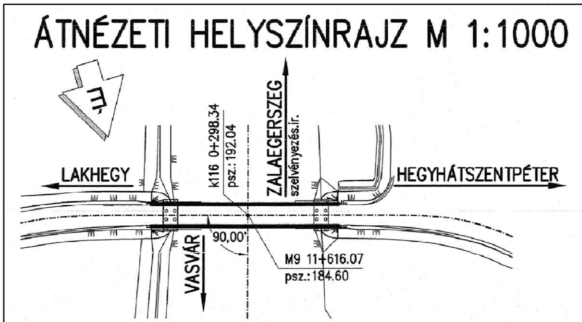
B.116 j. aluljáró a K116 J. önkormányzati út alatt
