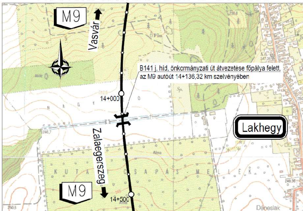
B.141 j. híd, önkormányzati út átvezetése főpálya felett, az M9 autótút 14+136,32 km szelvényében – Forrás: Hídépítés engedélyezési terv, Készítette: Vasvár-Zalaegerszeg Konzorcium
