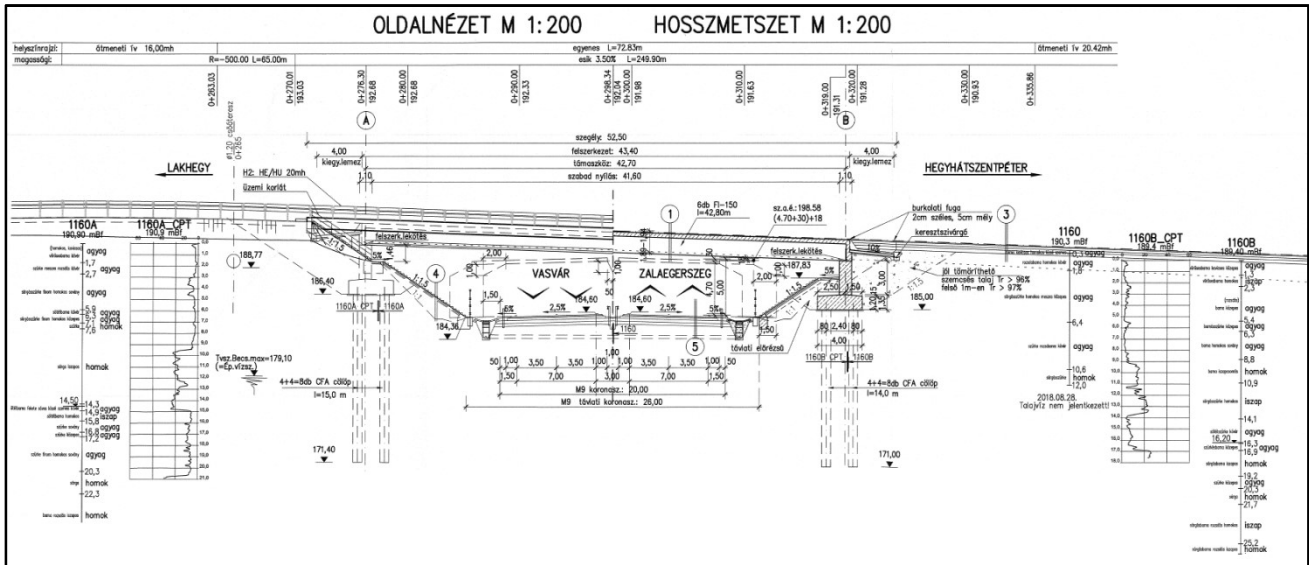
B.116 j. aluljáró a K116 J. önkormányzati út alatt Forrás: Hídépítés engedélyezési terv, Készítette: Vasvár-Zalaegerszeg Konzorcium
