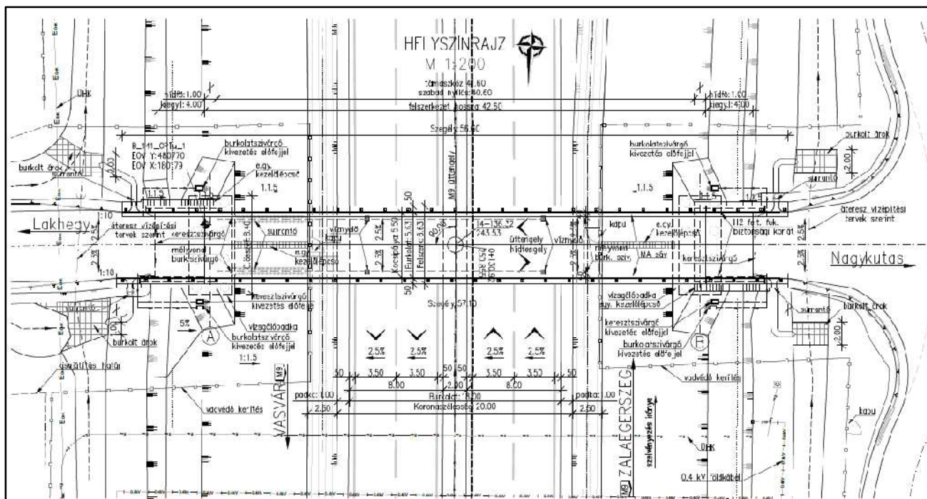
B.141 j. híd, önkormányzati út átvezetése főpálya felett, az M9 autópálya 14+136,32 km szelvényében – Forrás: Híddépítés engedélyezési terv, Készítette: Vasvár-Zalaegerszeg Konzorcium
