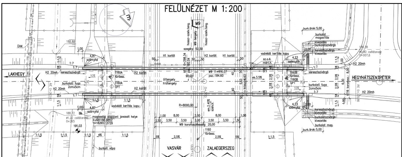
B.116 j. aluljáró a K116 J. önkormányzati út alatt – Forrás: Hídépítés engedélyezési terv, Készítette: Vasvár-Zalaegerszeg Konzorcium
